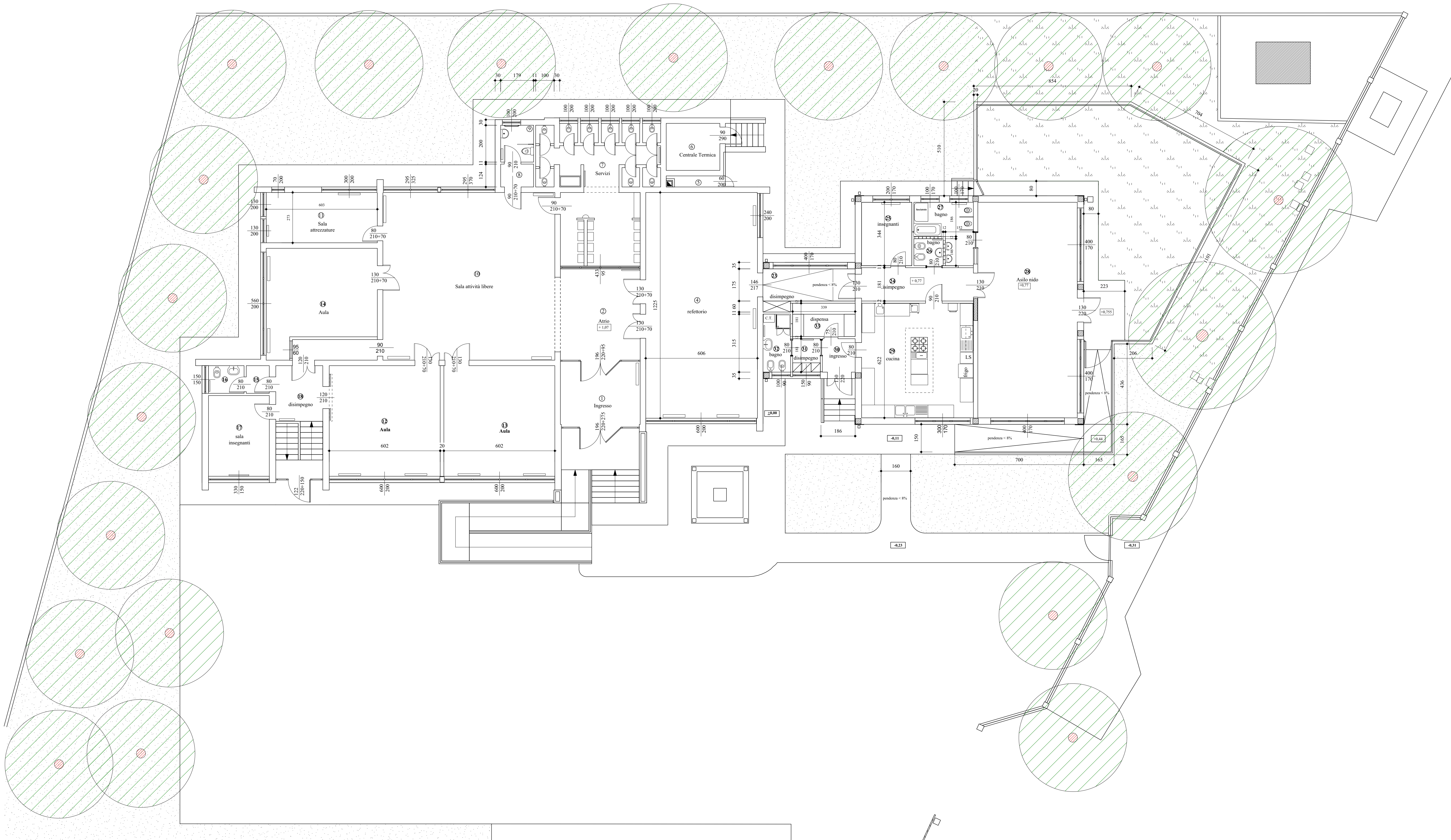
PLANIMETRIA GENERALE SCALA 1:100
